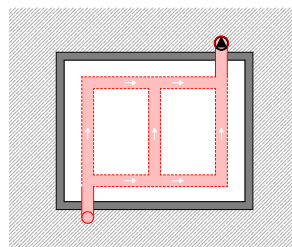
F.2 Pianta di posa di un drenaggio tipo con estrazione attiva
