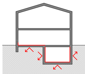
F.1 Parti dell'involucro a rischio di infiltrazioni
