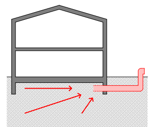
F.4 Sezione pozzo esterno
